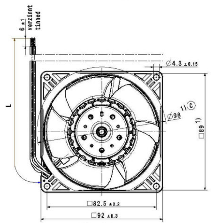
Vorderansicht Maßstab: 1:1 front view scale: 1:1
