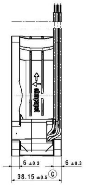
Seitenansicht links Maßstab: 1:1 side view left scale: 1:1
