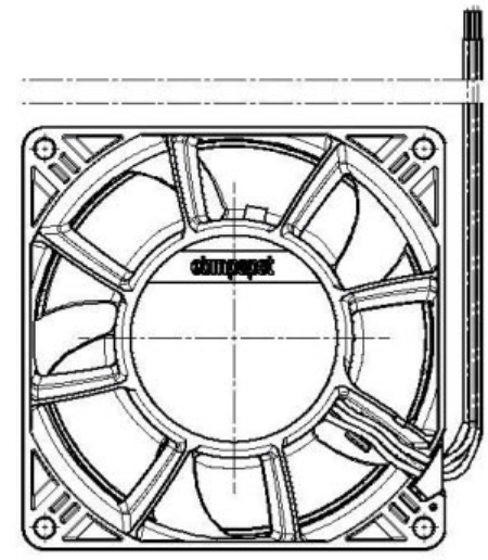
Rückansicht Maßstab: 1:1 back view scale: 1:1
