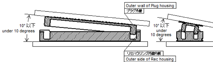
△ 図-2 外壁合せによる嵌合 Figure-2 Mating aligning to outer wall of housings (Acceptable)
