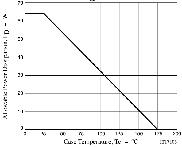
P_D - T_c
