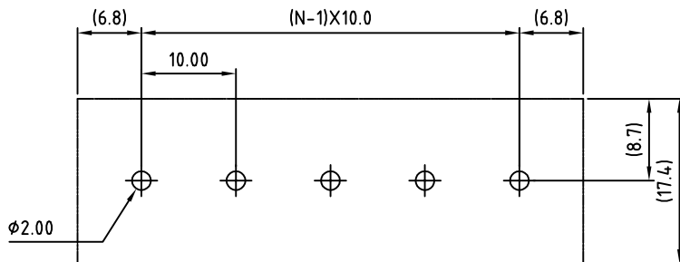
P.C.B LAYOUT
