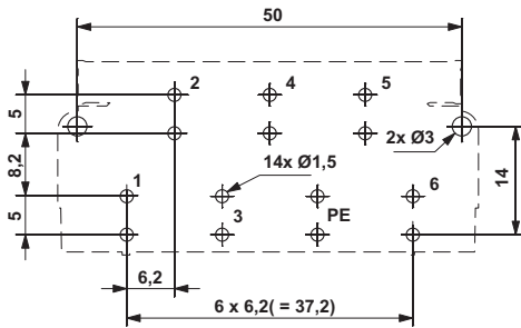
Drilling diagram: DC-...PCB-180
