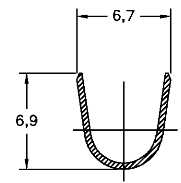
SECÇÃO B-B SECTION
