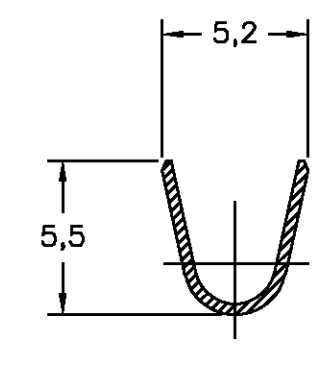
SECÇÃO A-A SECTION
