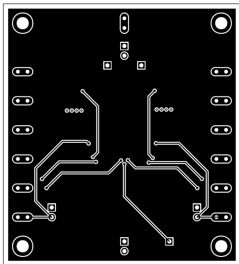
Layout—Inner Layer 1
