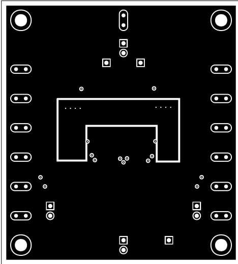
PCB Layout—Inner Layer 2
