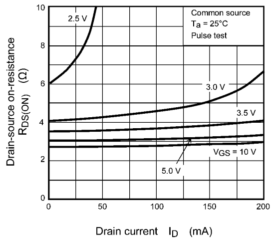
Fig. 7.4 R_{DS(ON)} - I_D
